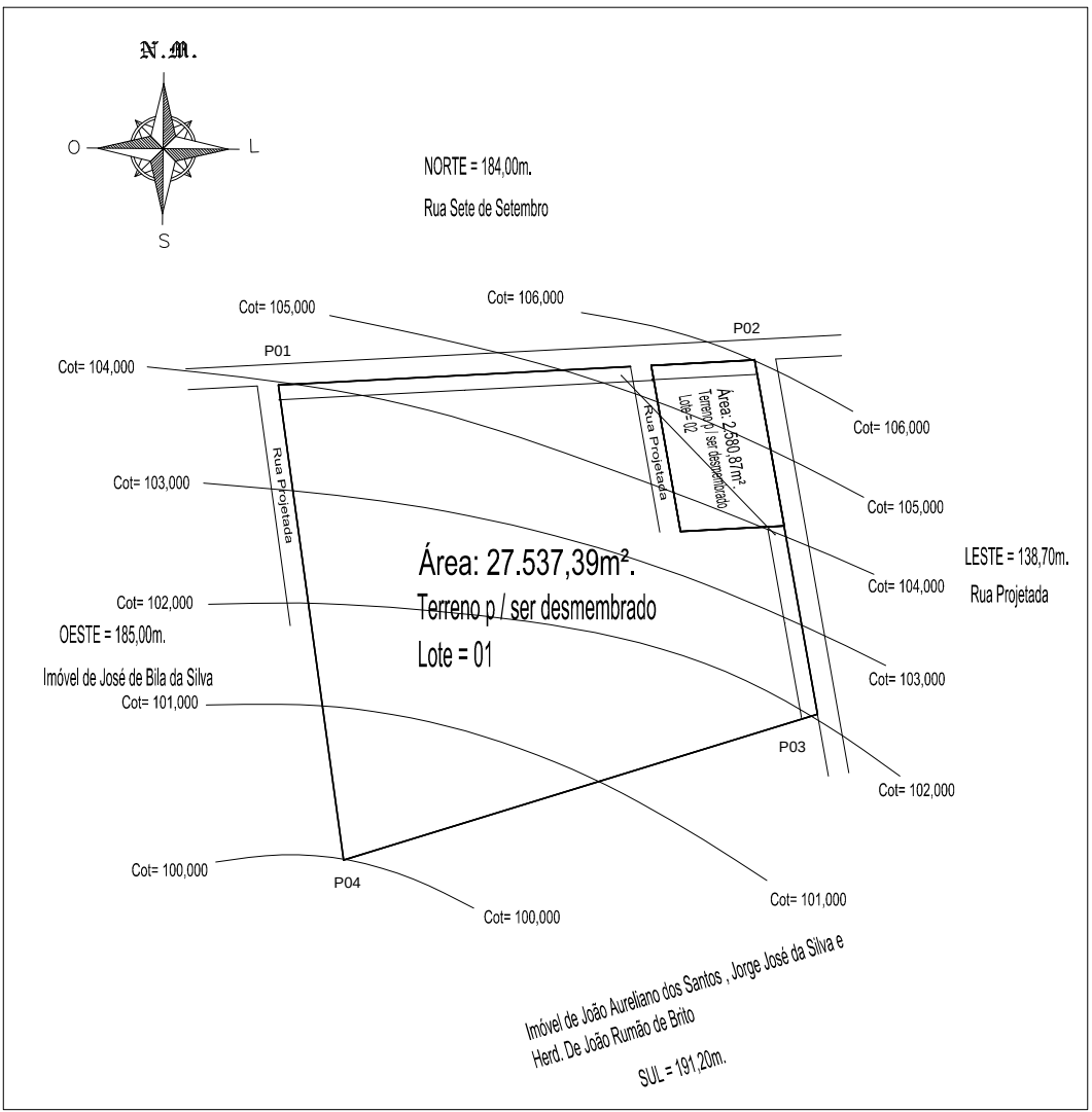
PLANTA SITUAÇÃO
